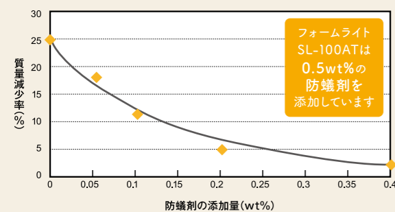
防蟻剤の添加量と質量減少の関係(自社評価法による)
