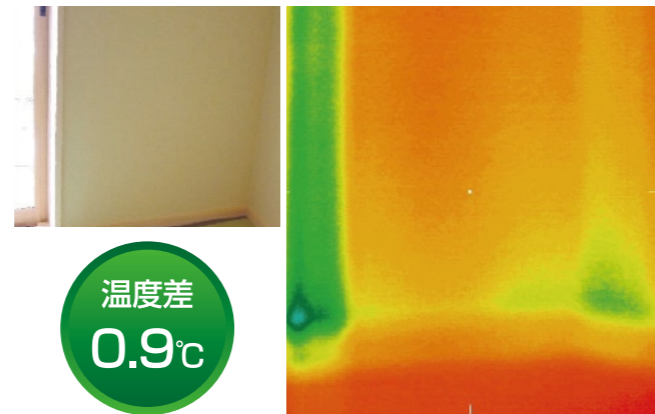
マシュマロ断熱は構造材(柱・土台)に接着をするため、冷気の侵入が無く、温度差が小さい。
