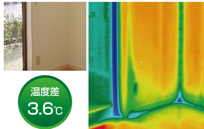
断熱材と構造材(柱・土台)のわずかな隙間から冷気が壁内に侵入しているため、温度差が大きい。
